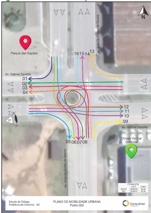
Figura 10: CPM-P002 – Croqui de Movimentos.
