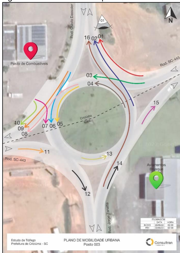
Figura 13: CPM-P003 – Croqui de Movimentos.
